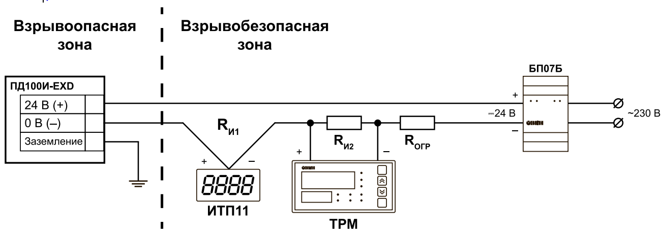
Рисунок 7.8 – Вариант схемы подключения ОВЕН ПД100И-EXD (модель 1х5)
