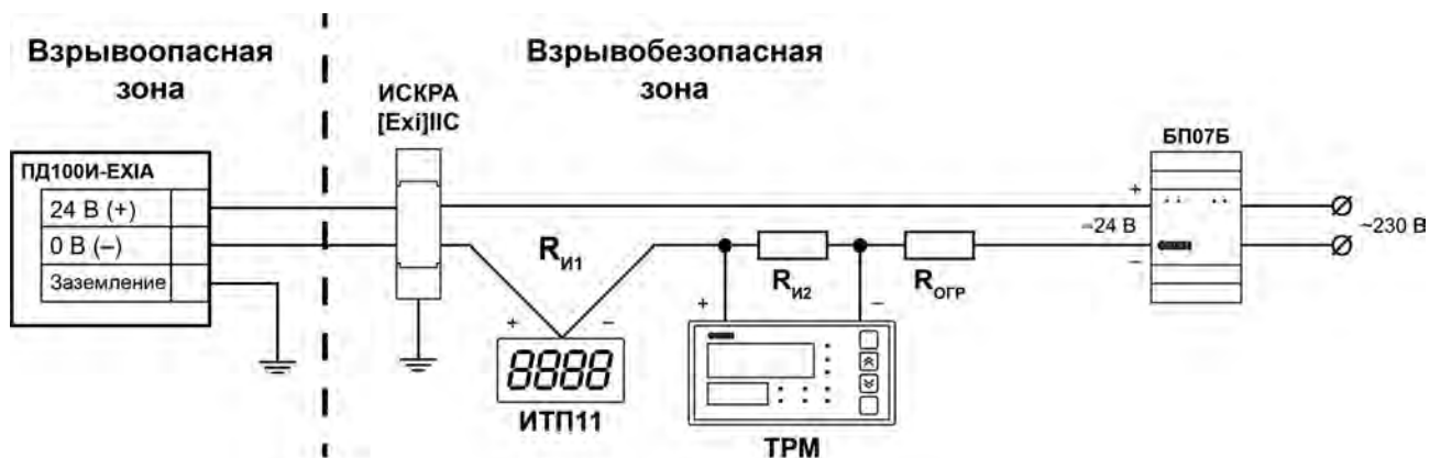
Рисунок 7.7 – Вариант схемы подключения ОВЕН ПД100И-EXI (модели 1х1, 1х7, 8х1)
