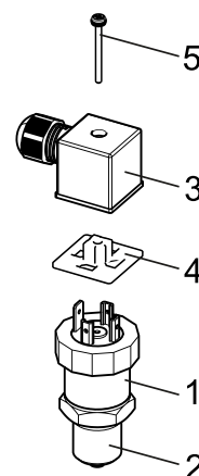
Рисунок 5.1 – Конструкция моделей 1х1 и 8х1
